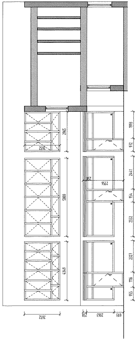
Pohľad od parkoviska 1 : 100
